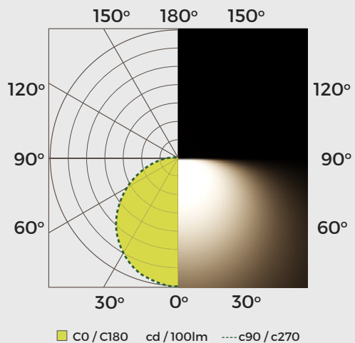
LPB24WD3KSS-MX2 - 30-40-50W - 3000K Intensidad lumínica
