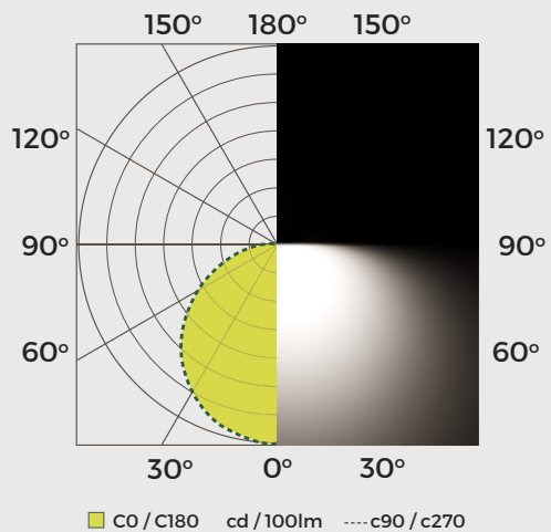
LPB24WD3KSS-MX2 - 30-40-50W - 5000K Intensidad lumínica
