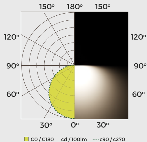
LPB24WD3KSS-MX2 - 30-40-50W - 4000K Intensidad lumínica
