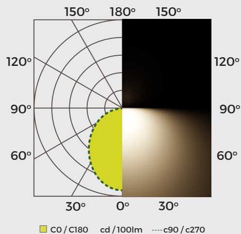
LPESQ18W18L3K-MX - 18W, 3000K Intensidad lumínica
