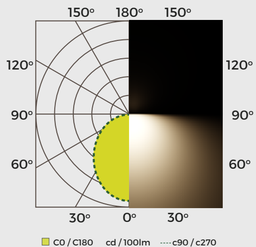
LPESQ24W24L3K-MX - 24W, 3000K Intensidad lumínica
