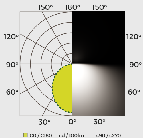
LPESQ24W24L3K-MX - 24W, 5000K Intensidad lumínica
