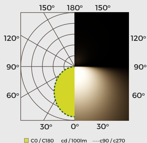
LPE18W18L3K-MX - 18W, 3000K Intensidad lumínica
