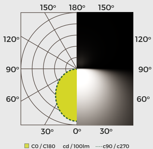
LPES24W24L3K-MX - 24W, 5000K Intensidad lumínica
