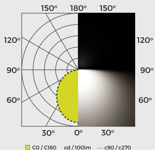
LPE12W12L3K-MX - 12W, 5000K Intensidad lumínica
