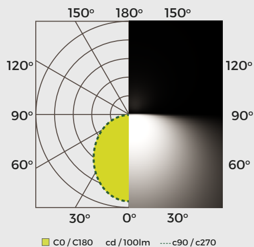
LPESQ18W18L3K-MX - 18W, 5000K Intensidad lumínica
