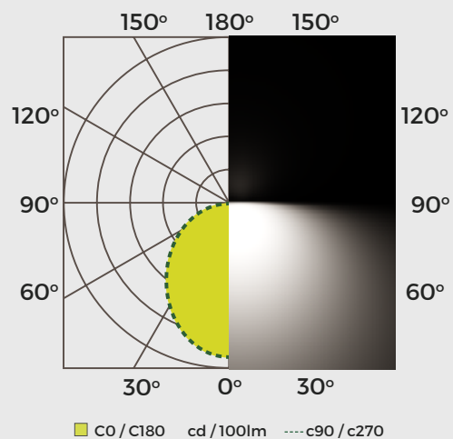
LPE18W18L3K-MX - 18W, 5000K Intensidad lumínica
