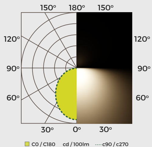
LPE12W12L3K-MX - 12W, 3000K Intensidad lumínica
