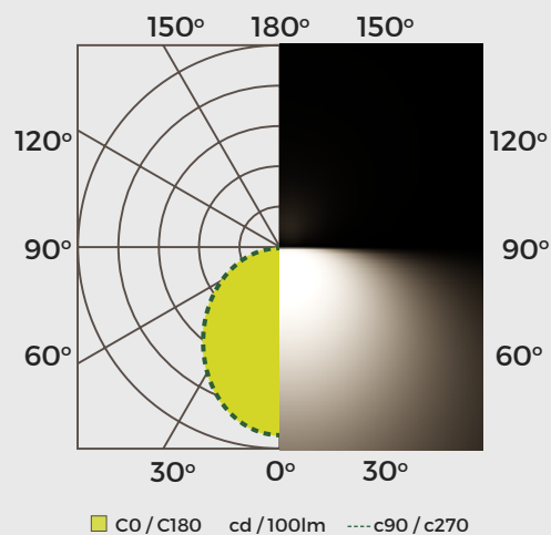
LPESQ24W24L3K-MX - 24W, 4000K Intensidad lumínica
