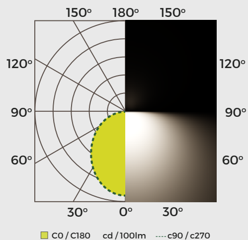
LPES24W24L3K-MX - 24W, 4000K Intensidad lumínica
