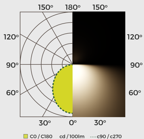
LPES24W24L3K-MX - 24W, 3000K Intensidad lumínica
