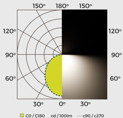
LPE18W18L3K-MX - 18W, 4000K Intensidad lumínica
