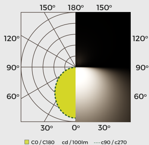
LPE12W12L3K-MX - 12W, 4000K Intensidad lumínica
