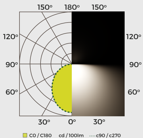
LPESQ18W18L3K-MX - 18W, 4000K Intensidad lumínica
